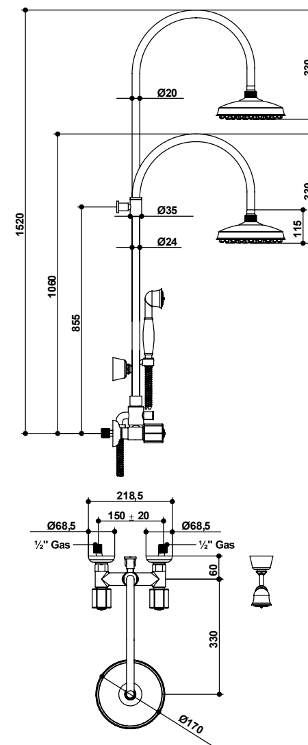
11537/D FLEUR BLANC 12537/D FLEUR NOIR Gruppo doccia esterno con tubo, soffione e set doccia duplex External shower mixer with tube, shower head and shower set duplex
