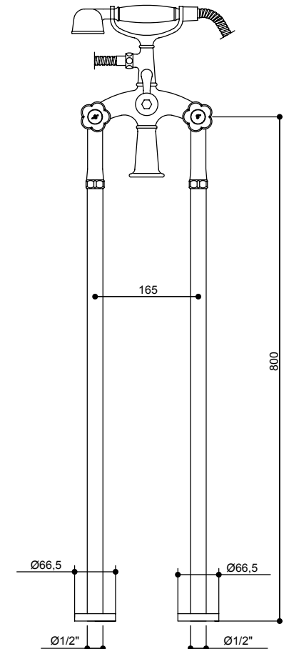
11528 FLEUR BLANC 12528 FLEUR NOIR Gruppo vasca esterno su colonnate da terra con set doccia External bath and shower mixer to the floor with shower set
