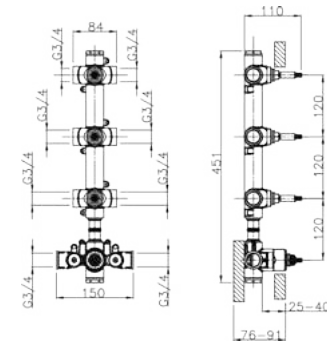
ZA 01V300 Parte Incasso Termostatico 3 Funzioni 3-Function Thermo Concealed Part Partie Encastrée Thermo 3 Fonctions
