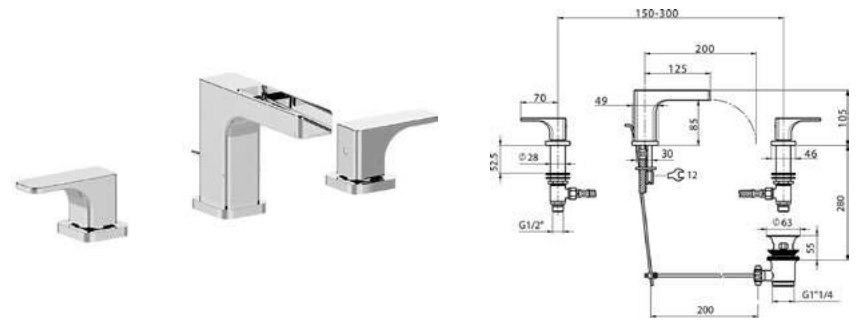
CU 0C1020 Batteria Lavabo Cascata Waterfall Basin Set Lavabo 3 Trou Cascade
