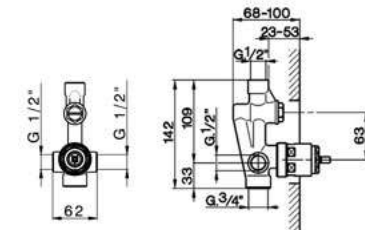
ZA 004211 Parte Incasso Monocomando 2 Uscite 2-Outlet Mixer Concealed Part Partie Encastrée Mitigeur 2 Sorties
