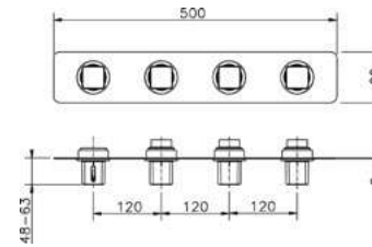
CU 01R300 Parte Esterna Termostatico 3 Funzioni 3-Function Thermo Exposed Part Partie Décor Thermo 3 Fonctions
