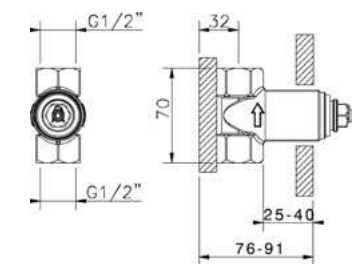
ZA 003340 Parte Incasso Rubinetto 1/2" 1/2" Stopvalve Concealed Part Partie Encastrée Robinet 1/2"
