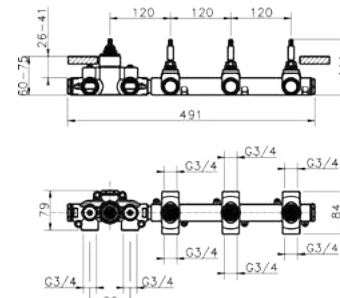
ZA 01R300 Parte Incasso Termostatico 3 Funzioni 3-Function Thermo Concealed Part Partie Encastrée Thermo 3 Fonctions
