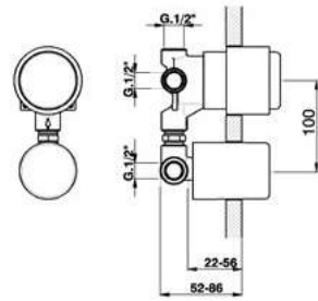
ZA 000280 Parte Incasso Monocomando 3 Uscite 3-Outlet Mixer Concealed Part Partie Encastrée Mitigeur 3 Sorties
