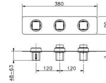
CU 01R200 Parte Esterna Termostatico 2 Funzioni 2-Function Thermo Exposed Part Partie Décor Thermo 2 Fonctions
