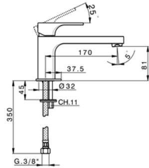
CU 001541 Monocomando Lavabo Basin Mixer Mitigeur Lavabo
