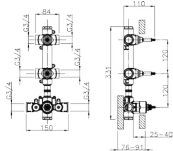
ZA 01V200 Parte Incasso Termostatico 2 Funzioni 2-Function Thermo Concealed Part Partie Encastrée Thermo 2 Fonctions
