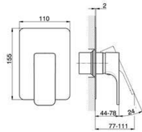
CU 003000 Parte Esterna Monocomando Doccia Shower Mixer Exposed Part Partie Décor Mitigeur Douche
