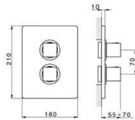
CU 007300 Parte Esterna Termostatico Doccia Thermo Shower Exposed Part Partie Décor Thermo Douche
