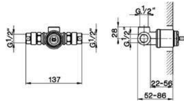
ZA 004310 Parte Incasso Monocomando Doccia con Silenziatori Shower Mixer Concealed Part with Noise Reducers Partie Encastrée Mitigeur Douche avec Silencieux
