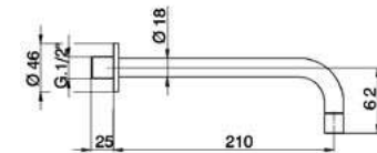
ZA 002250 Bocca di Erogazione Filler Spout Bec Verseur
