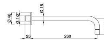
ZA 002251 Bocca di Erogazione Filler Spout Bec Verseur
