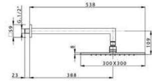
DS 013720 Braccio e Soffione Doccia Shower Arm & Head Bras et Tête de Douche
