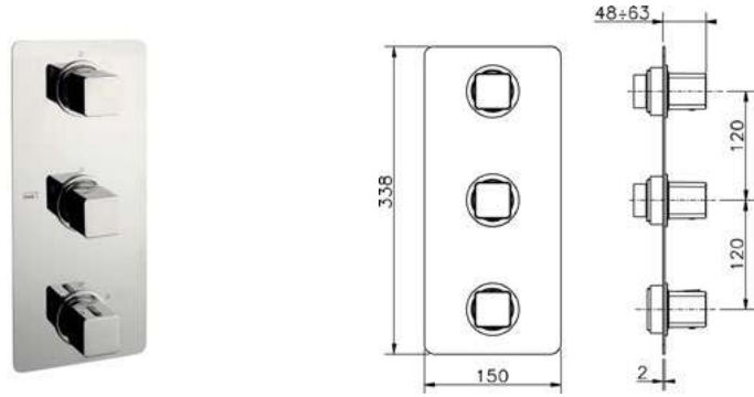
CU 01V200 Parte Esterna Termostatico 2 Funzioni 2-Function Thermo Exposed Part Partie Décor Thermo 2 Fonctions
