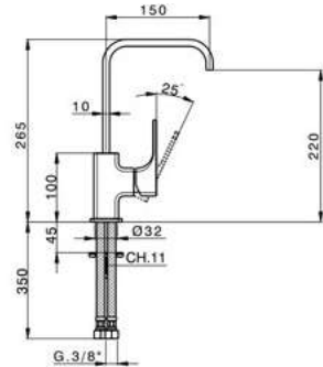
CU 000485 Monocomando Lavabo Basin Mixer Mitigeur Lavabo
