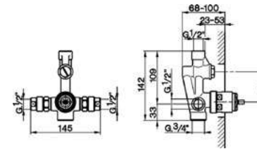
ZA 004210 Parte Incasso Monocomando 2 Uscite con Silenziatori 2-Outlet Mixer Concealed Part with Noise Reducers Partie Encastrée Mitigeur 2 Sorties avec Silencieux
