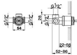
ZA 004311 Parte Incasso Monocomando Doccia Shower Mixer Concealed Part Partie Encastrée Mitigeur Douche
