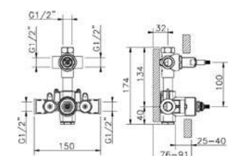
ZA 019201 Parte Incasso Termostatico 3 Uscite 3-Outlet Thermo Concealed Part Partie Encastrée Thermo 3 Sorties
