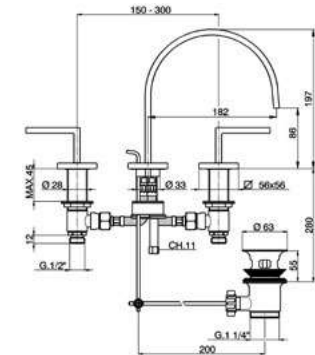
WA 001060 Batteria Lavabo Basin Set Lavabo 3 Trous
