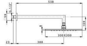
DS 013720 Braccio e Soffione Doccia Shower Arm & Head Bras et Tête de Douche
