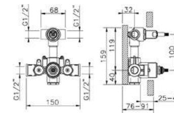
ZA 019101 Parte Incasso Termostatico 2 Uscite 2-Outlet Thermo Concealed Part Partie Encastrée Thermo 2 Sorties
